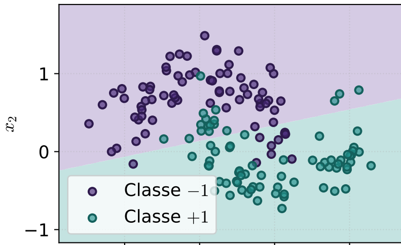
(a) Linéaire — acc. test = 0.88
