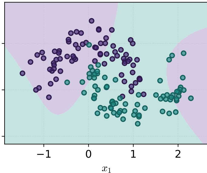
(d) Sigmoidale — acc. test = 0.68
